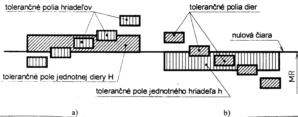
Uloženia v sústave jednotnej diery (a) a jednotného hriadeľa (b)
