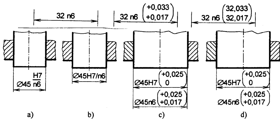
Zápis pomocou tolerančných značiek ISO na výkresoch zostáv
