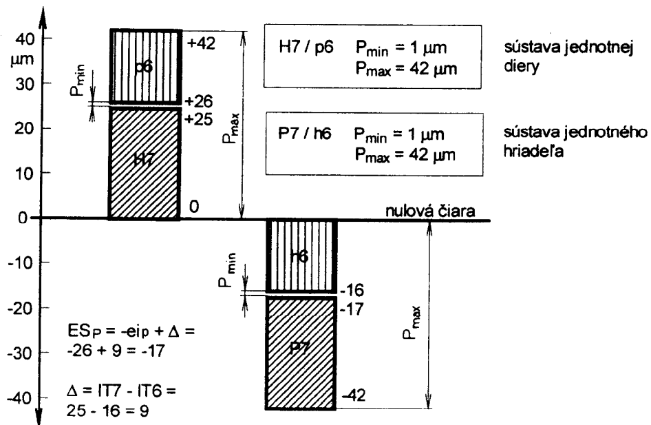
Prehľad polôh tolerančných polí hriadeľov a dier
