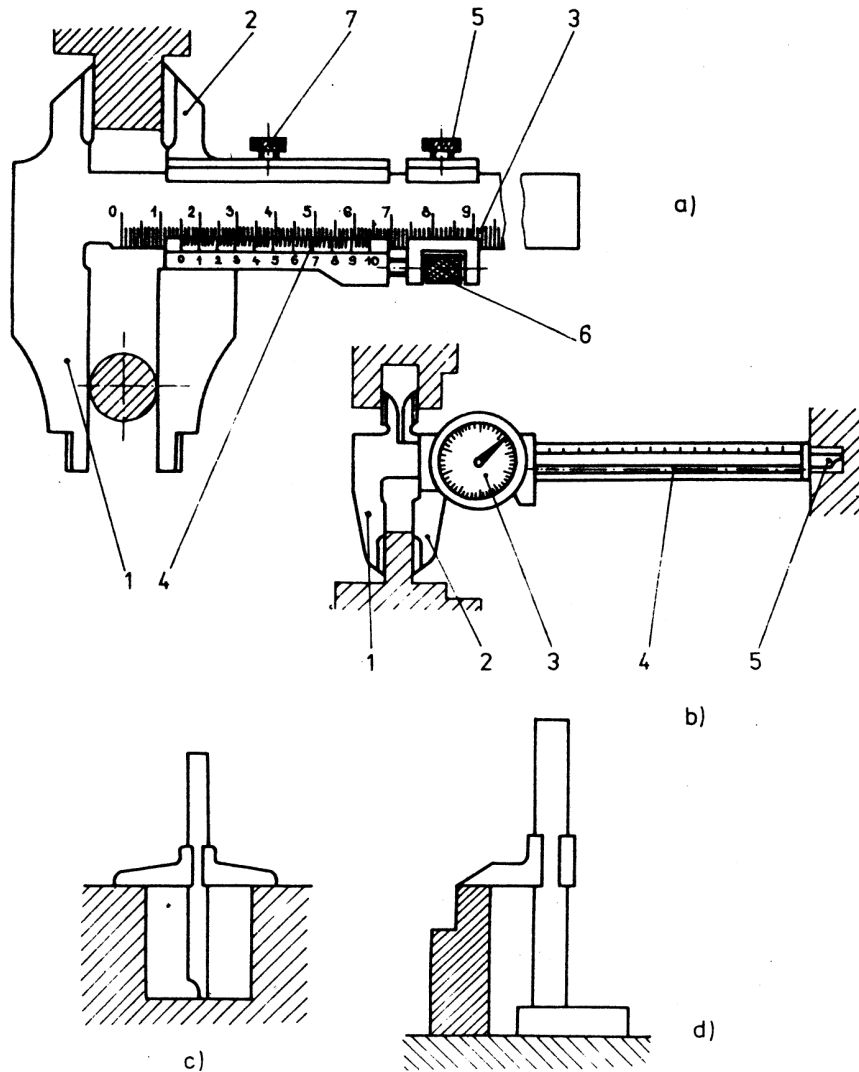
Čiarkované meradlá: a) základný typ posuvného meradla: 1 - pevná meracia čelust', 2 - pohyblivá meracia čelust', 3 - milimetrová stupnica, 4 - noniusová stupnica, 5 - zaistovacia skrutka jemného posuvu noniusa, 6 - jemný posuv noniusa, 7 - zaistovacia skrutka pohyblivej meracej čeluste; b) univerzálne posuvné meradlo s číselníkom: 1 - pevná meracia čelust', 2 - pohyblivá meracia čelust', 3 - číselník hodnôt, 4 - ozubená tyč prevodu ručičky číselníka, 5 - merací dotyk hĺbkomeru; c) hĺbkomer; d) výškomer
