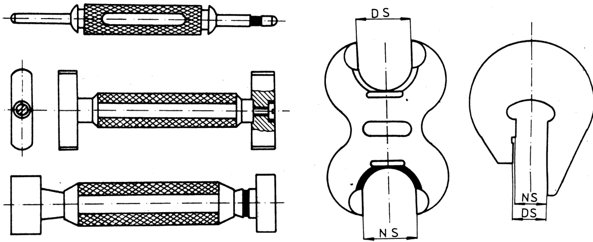
Príklady kalibrov pre meranie hriadel'ov: DS - dobrá strana, NS - nepodarková strana
