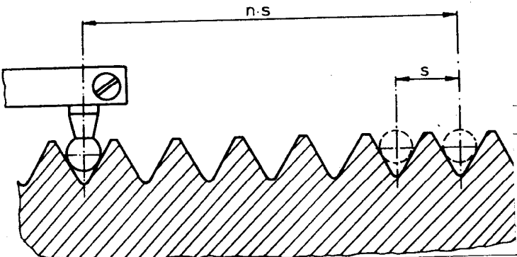
Princíp merania stúpania závitú skrutky dĺžkovým meracím prístrojom pomocou guľového dotyku
