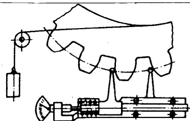
Schéma merania rozstupu na rozstupovej kružnici
