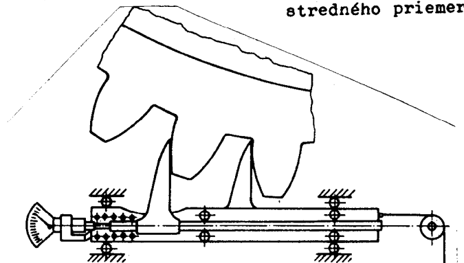
Schéma merania záberového rozstupu na univerzálnom prístroji na kontrolu ozubených kolies Zeiss
