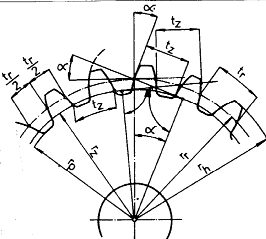
Čelné evolventné ozubenie
