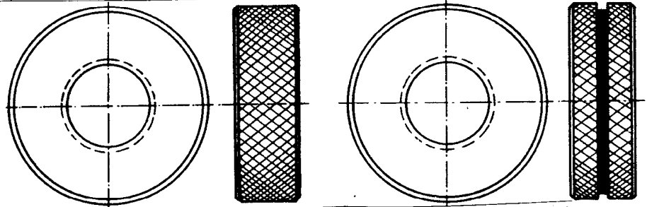
Medzné závitové krúžky: a) dobrý, b) nepodarkový
