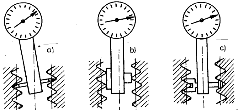
Meranie priemerov závitú matice: a) meranie veľkého priemeru, b) meranie malého priemeru, c) meranie stredného priemeru
