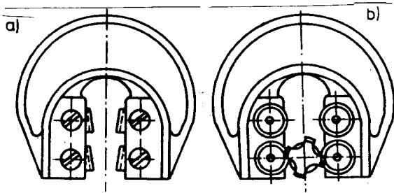
Medzné závitové strmeňové kalibre: a) hrebienkové, b) kladíčkové
