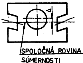
Odchýlka súmernosti od spoločnej roviny súmernosti
