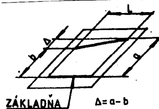
Odchýlka rovnobežnosti osí (priamok) v rovine
