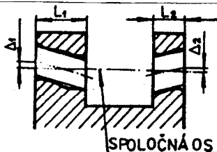
Odchýlka súosovosti od spoločnej osi
