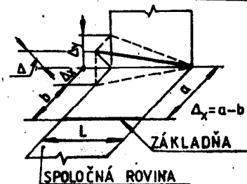
Odchýlka rovnobežnosti osi (priamok) v priestore
