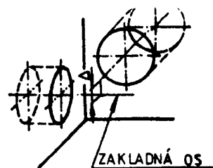
Odchýlka rôznobežnosti osí
