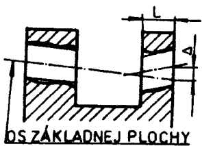
Odchýlka súosovosti od osi základnej plochy
