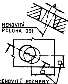
Odchýlka polohy prvku od menovitej polohy
