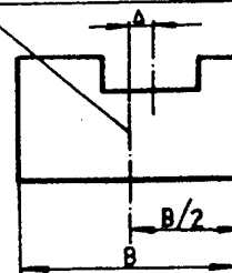
Odchýlka súmernosti od základnej roviny súmernosti
