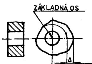
Obvodové hádzanie
