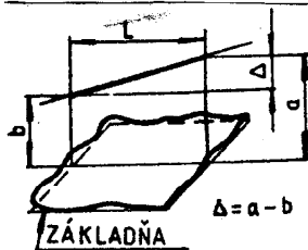
Odchýlka rovnobežnosti osi (priamky) s rovinou
