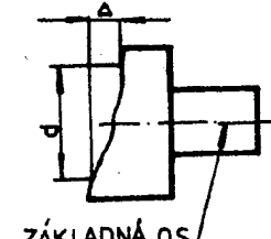
Čelné hádzanie
