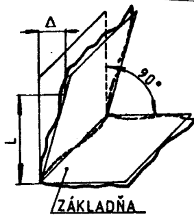
Odchýlka kolmosti
