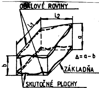
Odchýlka rovnobežnosti rovin
