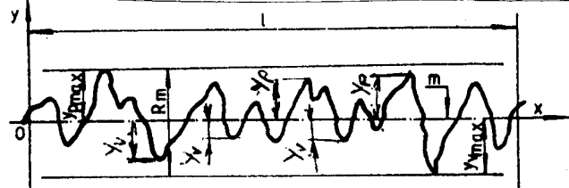
Výška najväčšieho výstupku a hĺbka najväčšej priehlbiny
