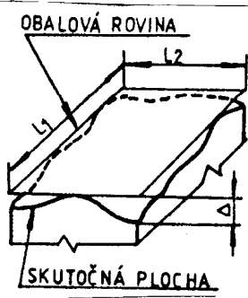
Odchýlka rovinnosti
