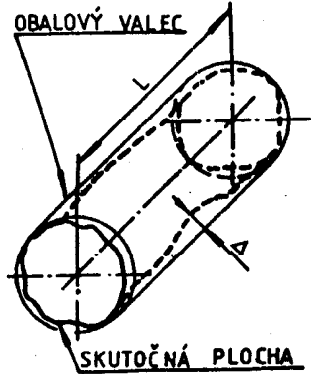
Odchýlka valcovitosti
