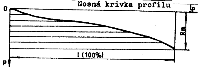
Stredná aritmetická odchýlka profilu
