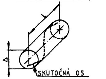
Odchýlka priamosti osi (čiary) v priestore
