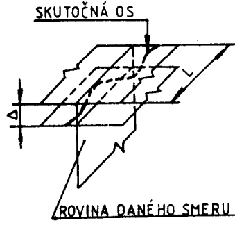
Odchýlka priamosti osi (čiary) v danom smere
