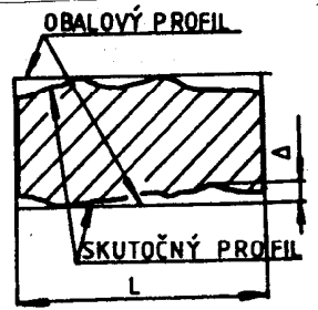
Odchýlka profilu pozdĺžneho rezu
