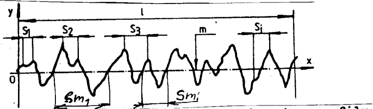
Rozstup miestnych výstupkov profilu
