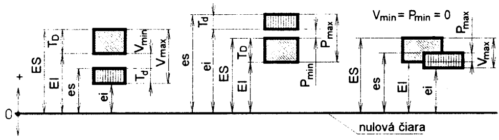
a) uloženie s vôľou
