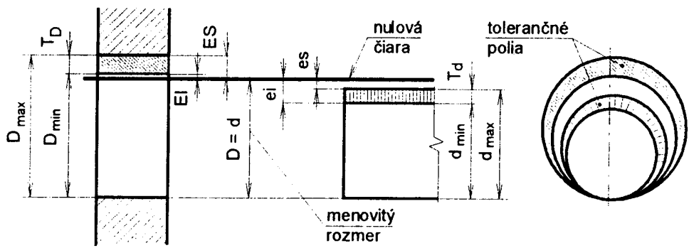
Tolerančné polia valcovej diery a valcového hriadeľa
