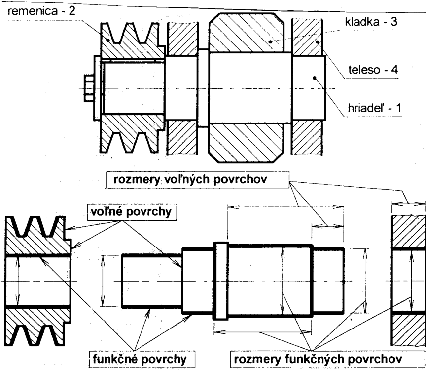
Funkčné a voľné povrchy súčiastok
